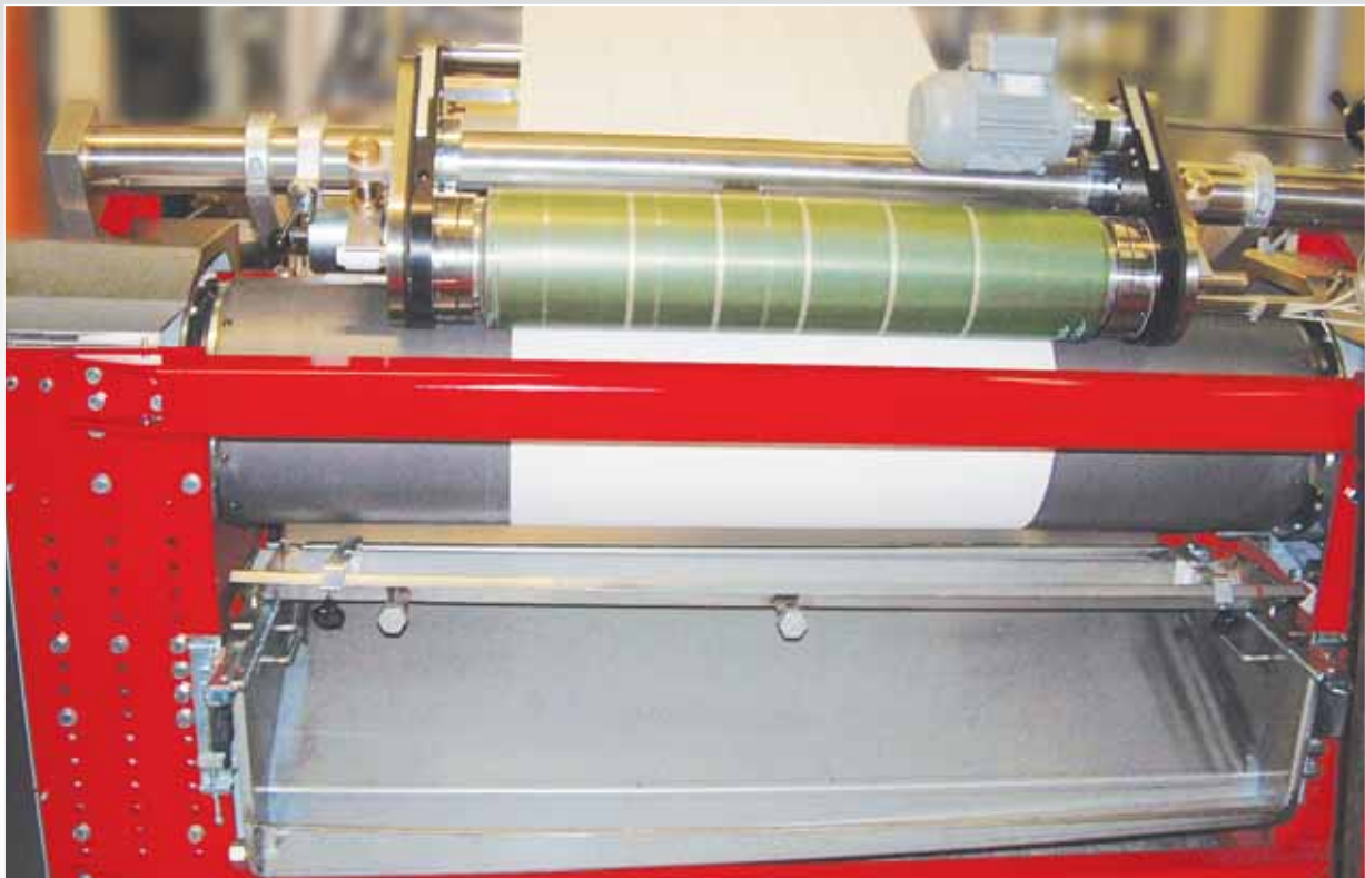
Beispiel: Produktion von Iridinstreifen auf Sicherheitspapier und EURO-Geldscheinen. Example: Production of iridescent stripes on safety paper and EURO-banknotes.
